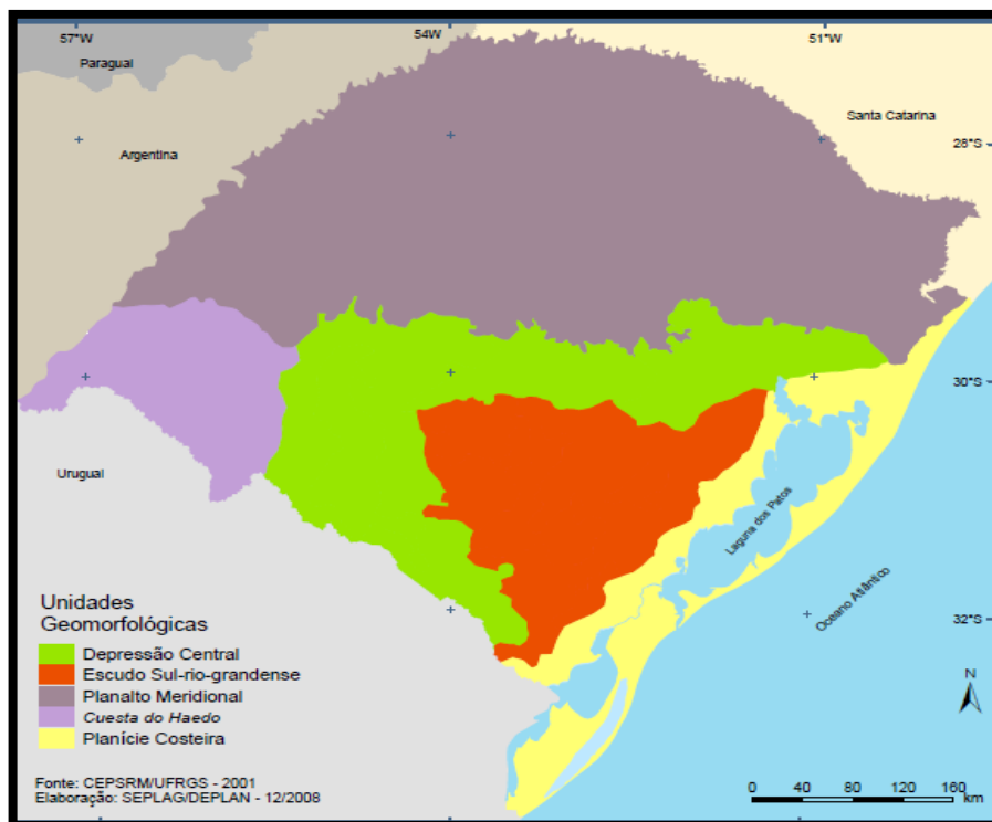
Figura 13: Províncias Geomorfológicas do Estado do Rio Grande do Sul.
