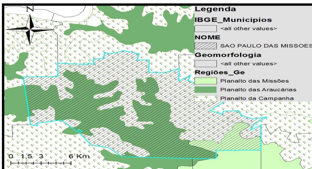
Figura 14: Geomorfologia do Município.
