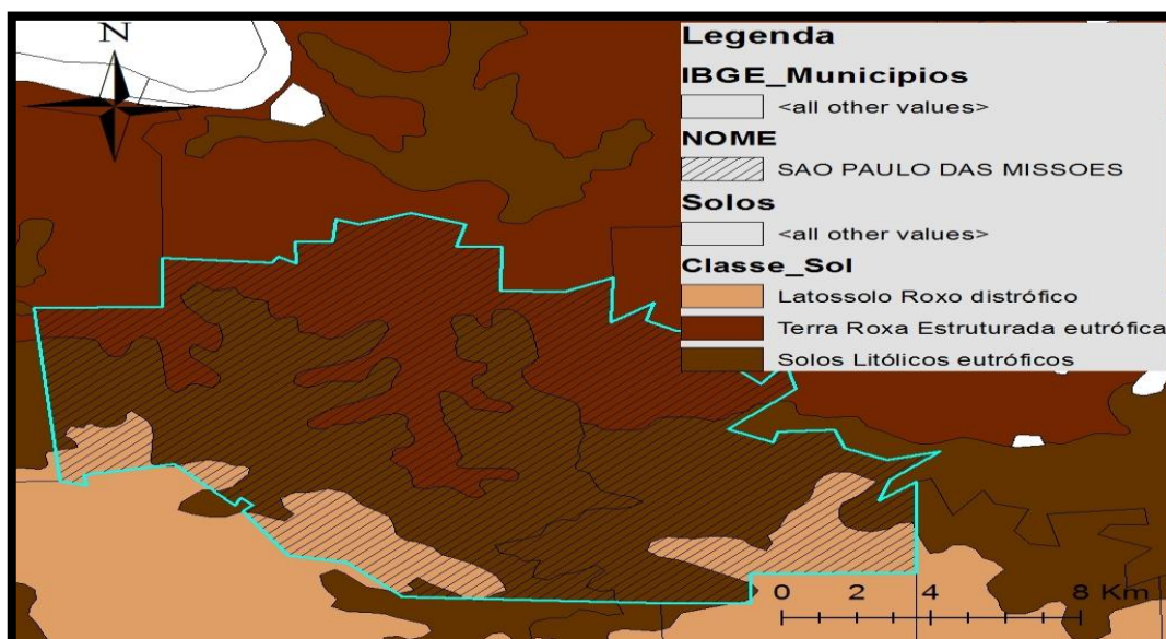
Figura 16: Solo do Município.
