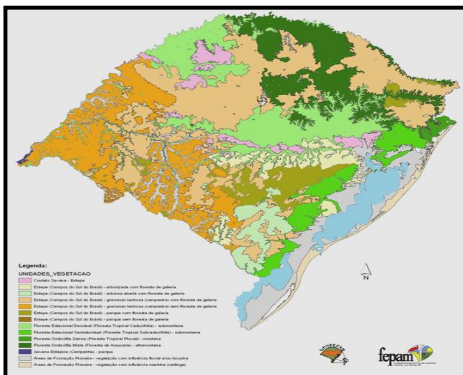
Figura 26: Unidades de Vegetação do Rio Grande do Sul.
