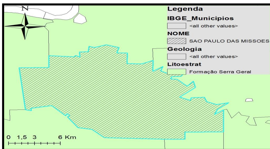
Figura 12: Geologia do Município.
