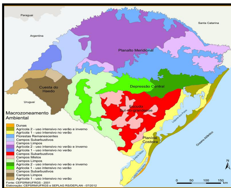
Figura 10: Regiões Fisiográficas do RS.
