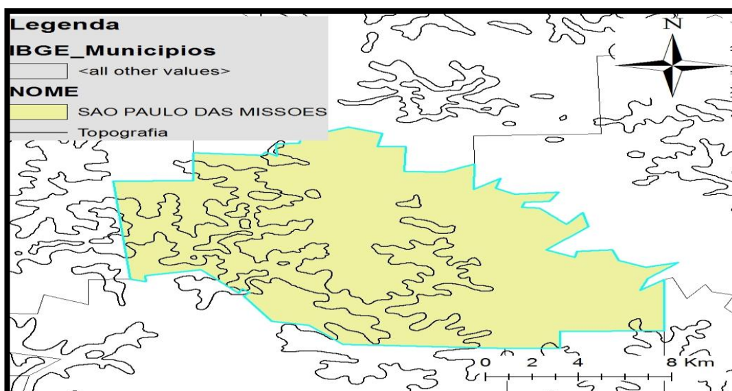
Figura 25: Topografia do Município.
